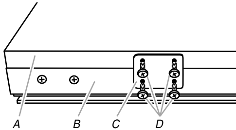
A. Panneau décoratif B. Porte C. Plaques décoratives (2) D. Vis à tête ronde (8)
