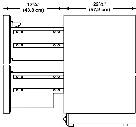
Dimensions de largeur de tiroir
